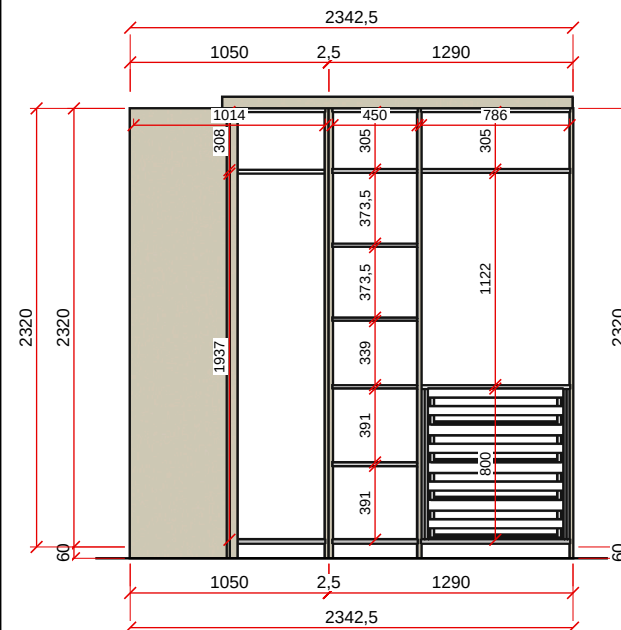
VISTA D - ESC. 1:40
