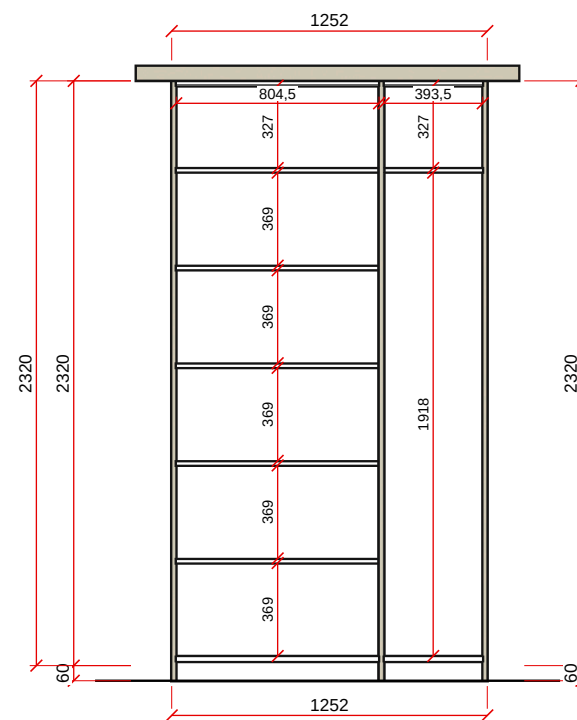
VISTA B - ESC. 1:30
